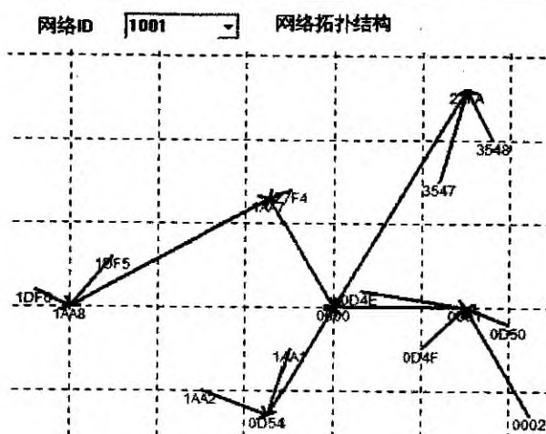
图3 网络ID为0X1001的网络拓扑结构图
