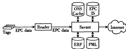
图2 EPC系统的基本组成
